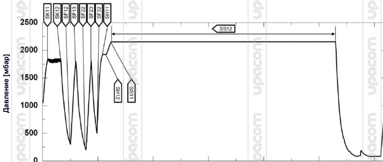
Диаграммы давление-время для Щадящая В, 121 °C и 1,1 бар
