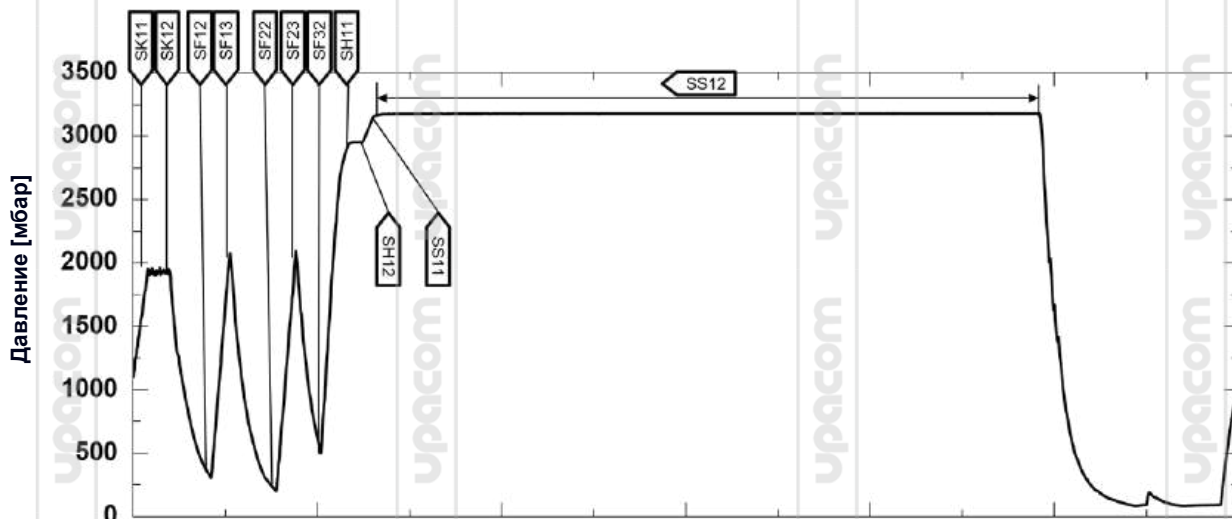
Диаграммы давление-время для Прион В, 134 °C и 2,1 бар
